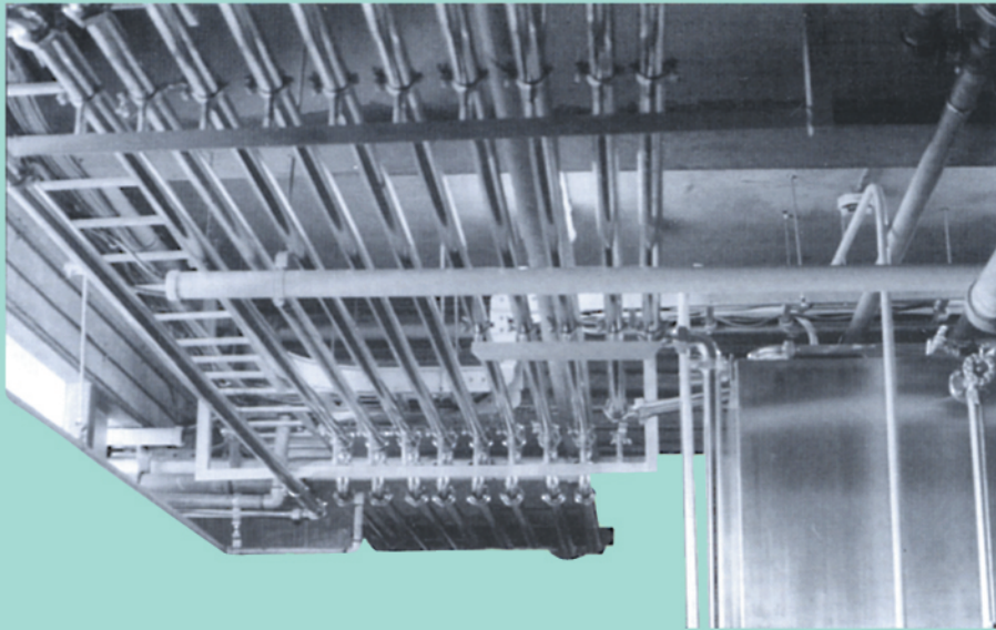
サニタリー配管 (一例)
