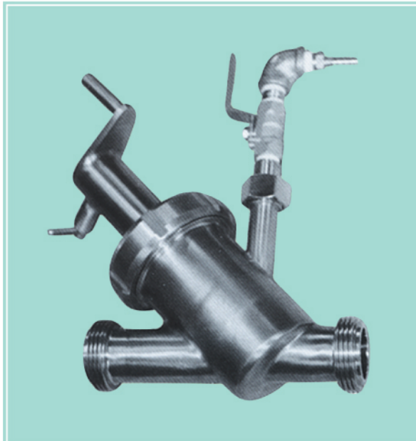
Y型ハンドバルブ (スチームノズル付)
