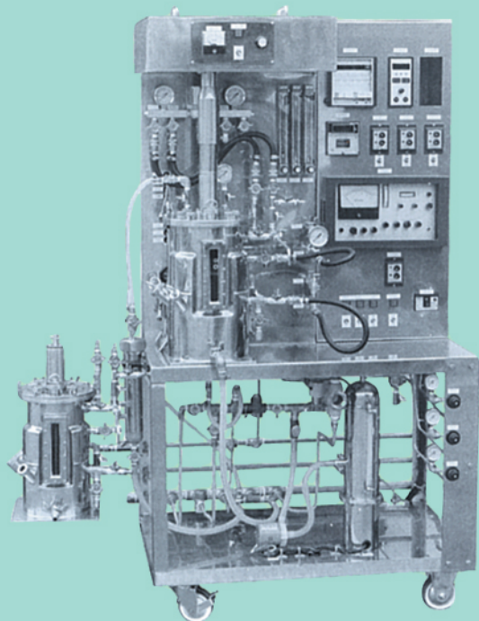
■ミニジャーファーメンター5ℓ～10ℓ兼用型
